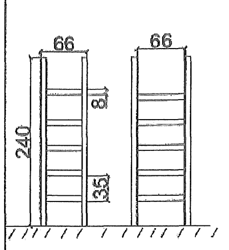
zobrazení žebříků přeazu
