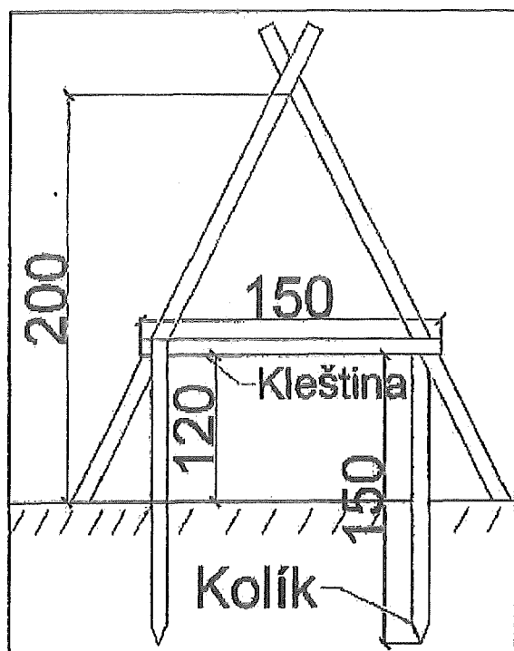
Bóční náčres zhotovení přeazu a
