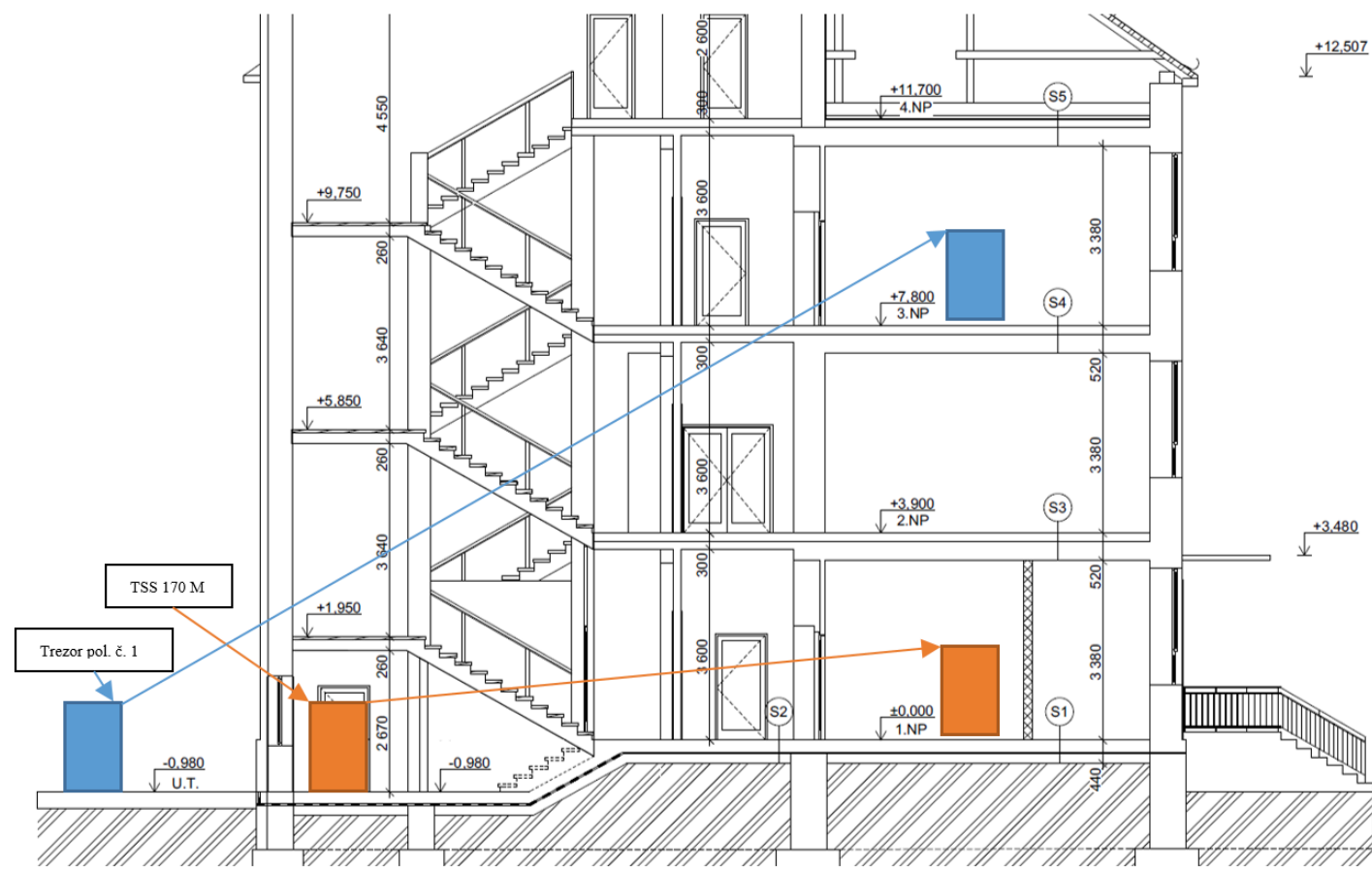
Položka č. 3 Situační plánek k instalaci trezorů na budově č. 3
