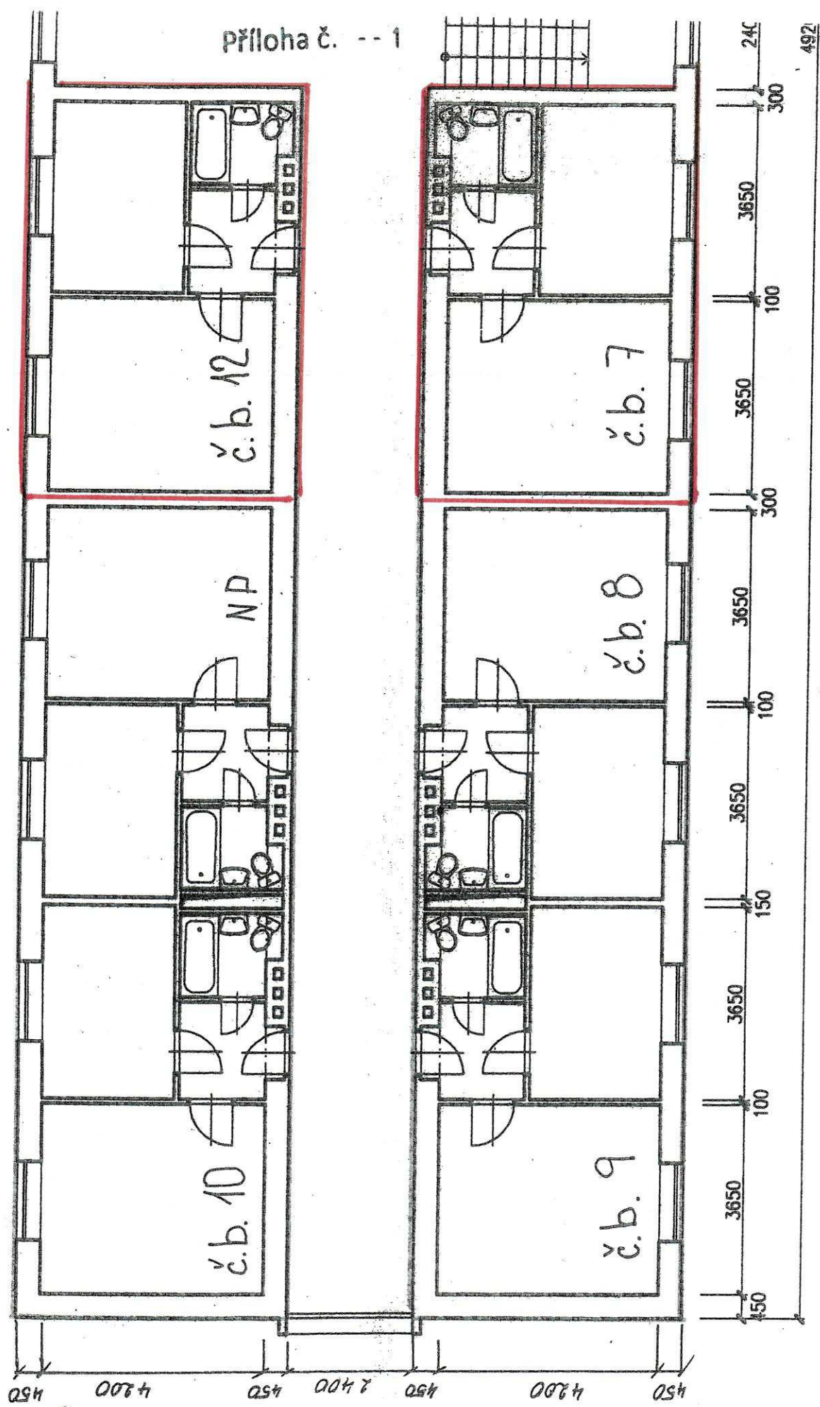
PŮDORYS 2.NP
