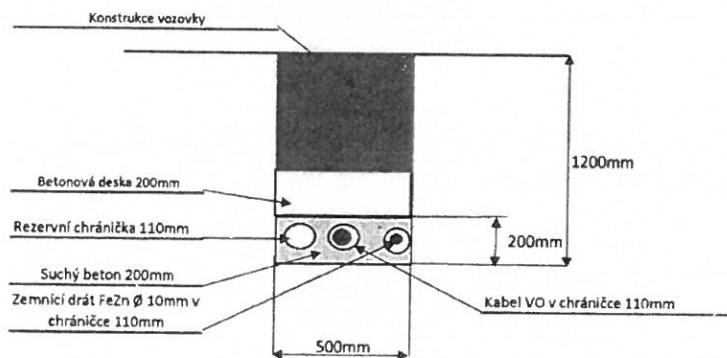
Vzorový řez uložení kabelu v chrániči pod vozovkou
