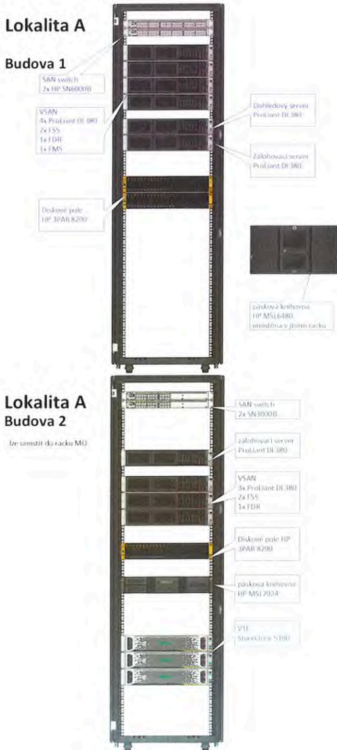
Příloha č. 1 Obrázek „Schéma zapojení v racku pro lokalitu A“ – 1 list
