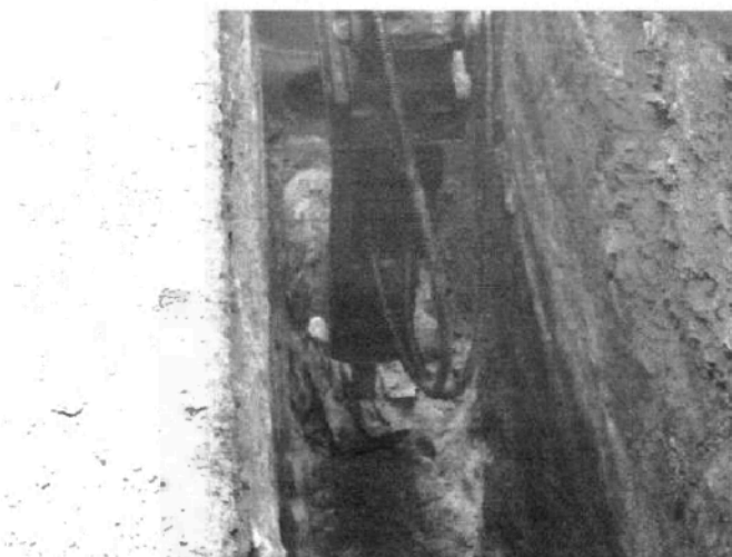
Obr. 4 – rozpojování hornin tř.7
