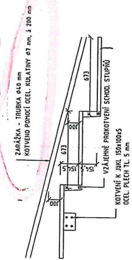
ROZVINUTÝ POHLED - VNĚJŠÍ M 1:20
