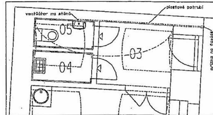
DETAIL TRASY VEDENÍ ODVĚTRÁNÍ WC 1:50
