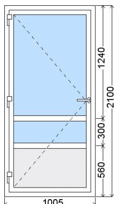
Vchodové dveře otvíravé ven - pohled exteriér
