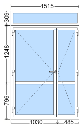
Vchodové dveře otvíravé ven - pohled exteriér
