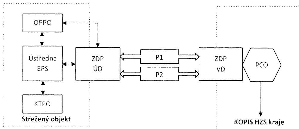
Schéma zařízení dálkového přenosu
