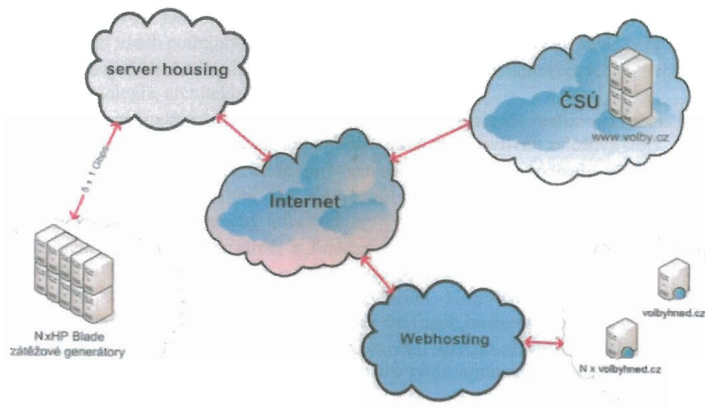
Obrázek 1: Architektura zátěžového testu
