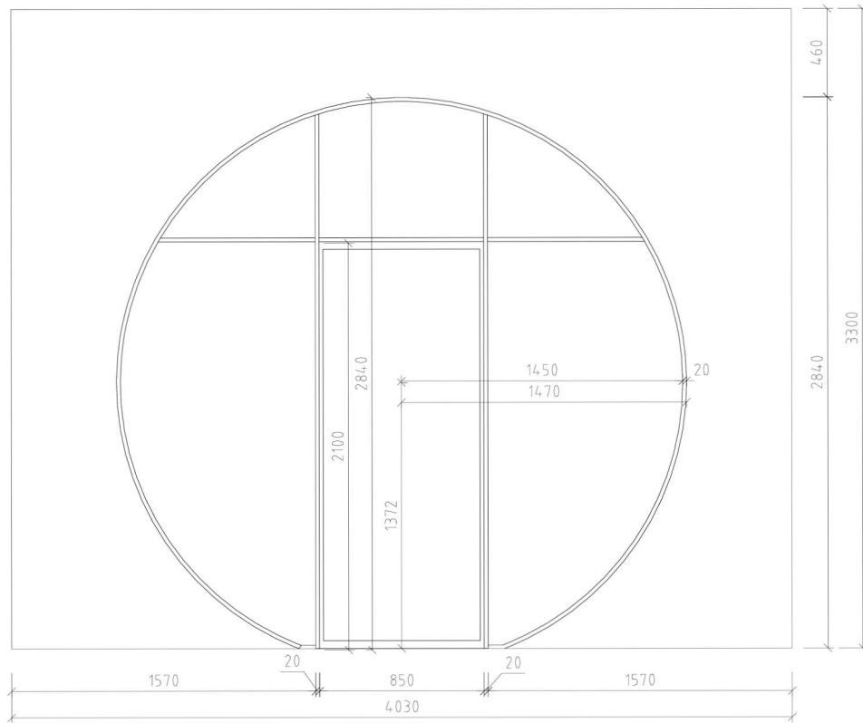
pohled A
