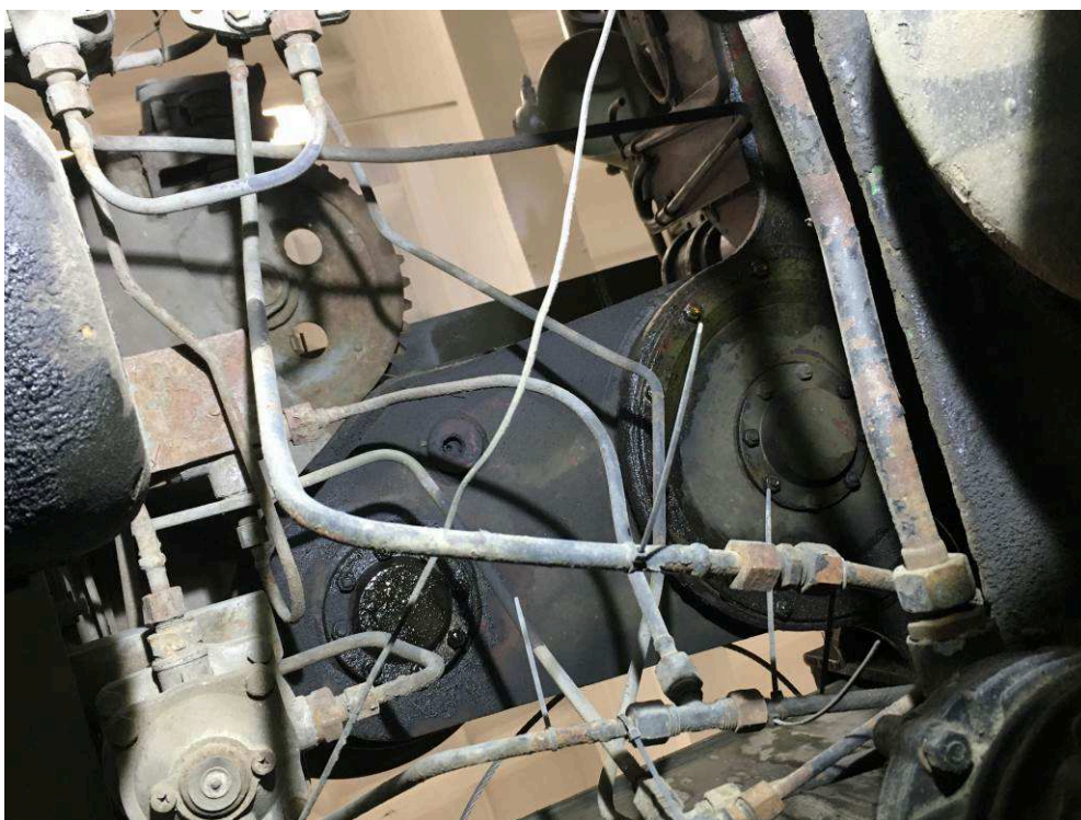
Foto č. 3 - Přetěsnění náhonu kuželových kol brzdy lana.
