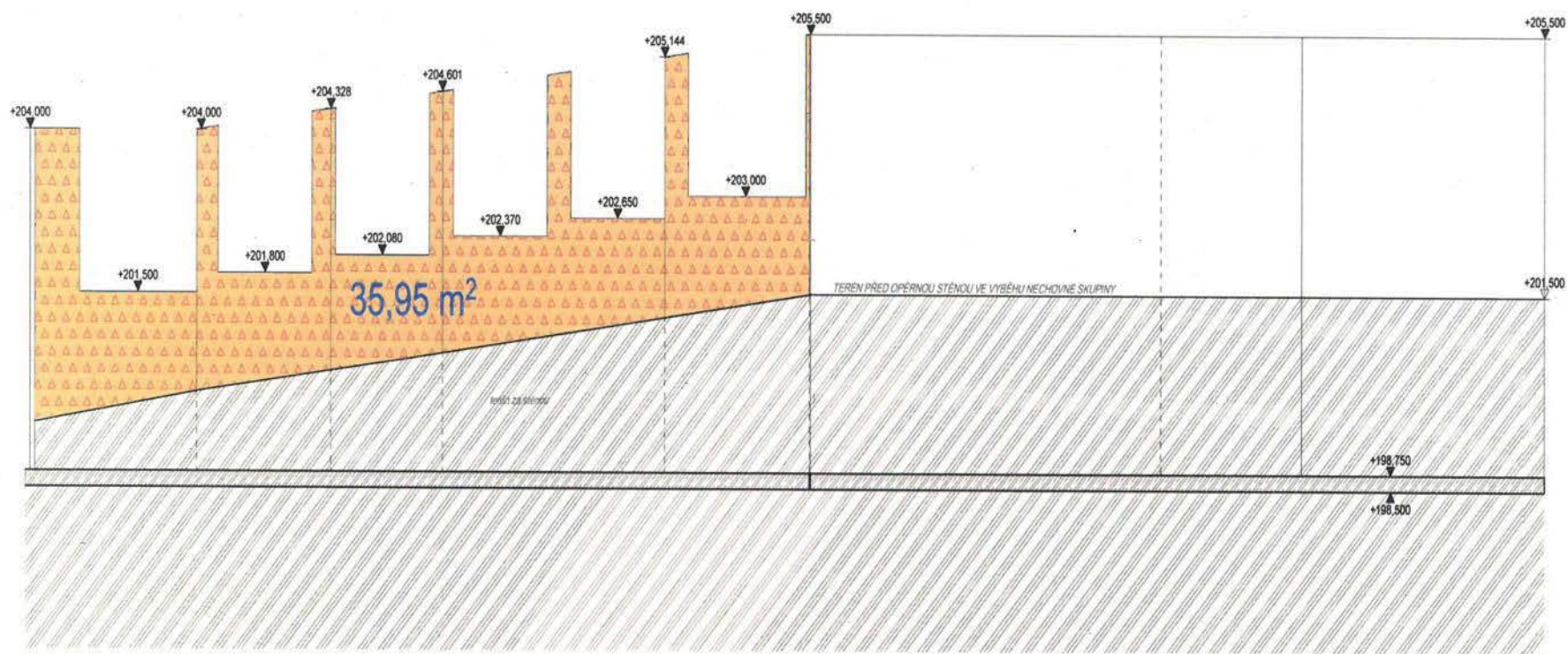
Výkresová příloha č. 1 k ZL č. 3 ze dne 14.7.2020_ vnitřní strana TRK 44, venkov.výběh nechov. skupiny, pavilon goril, ZOO Praha
