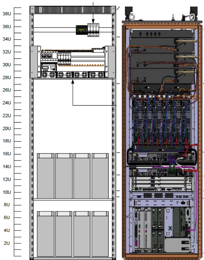
Obr. 4 sestava technologie
