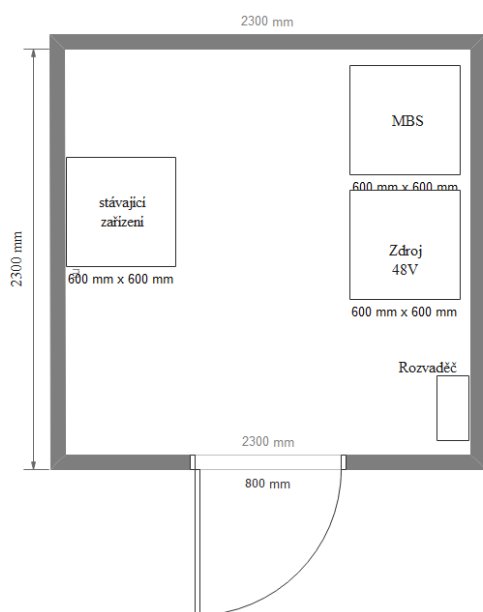
Obr 3. Umístění technologie v kontejneru
