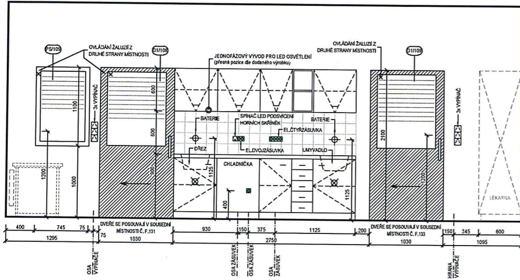
POHLED "C" - 1:25
