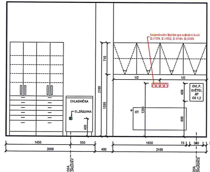
POHLED "D" - 1:25
