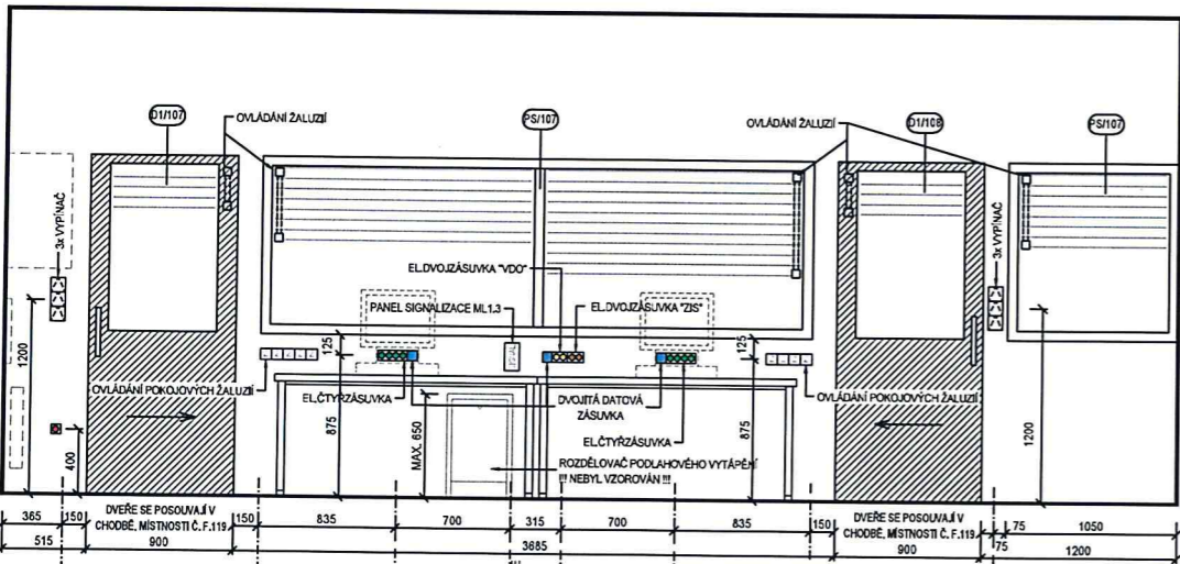
POHLED "C" - 1:25
