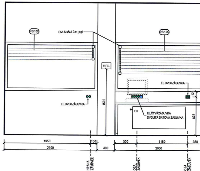
POHLED "D" - 1:25
