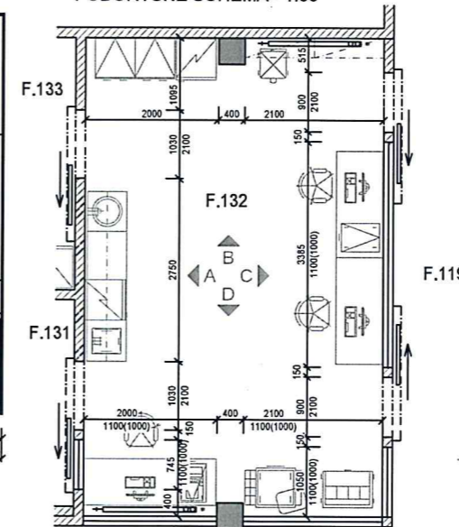
PŮDORYSNÉ SCHÉMA - 1:50
