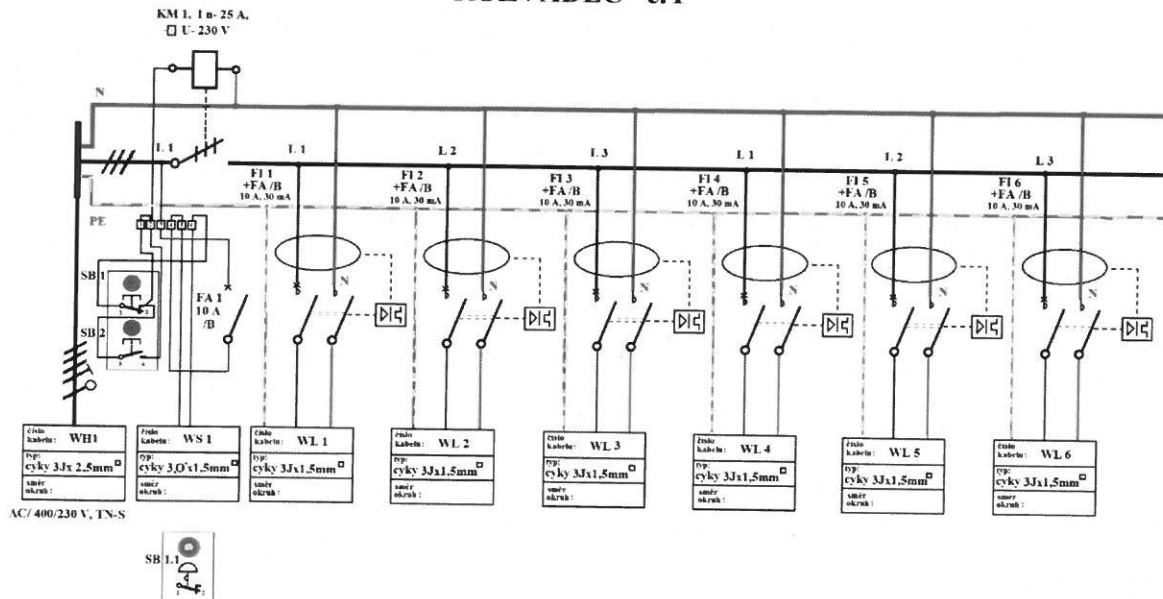
Schéma vybavení podružného rozvaděče v demonstračním stole
