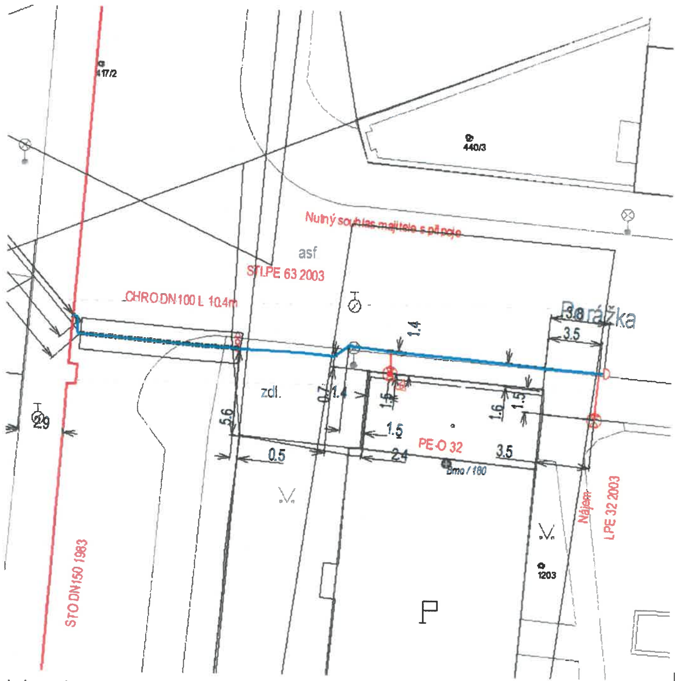
úsek plynovody
