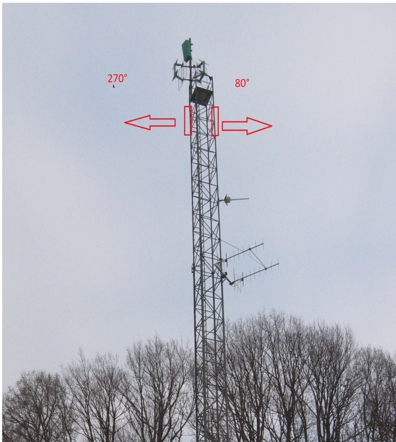
Obr. 3 návrh umístění antén
