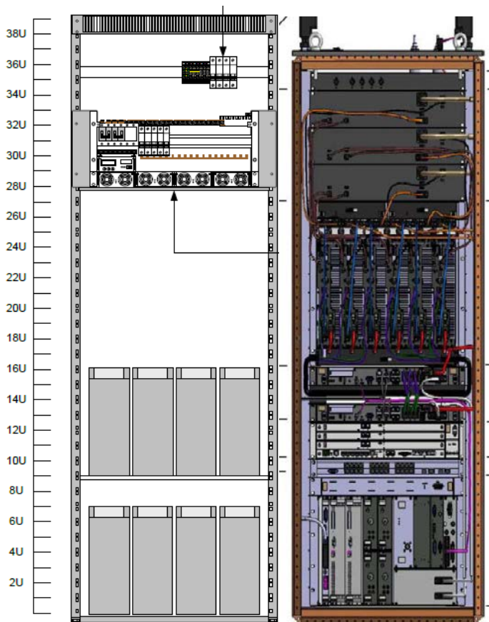
Obr. 2 sestava technologie
