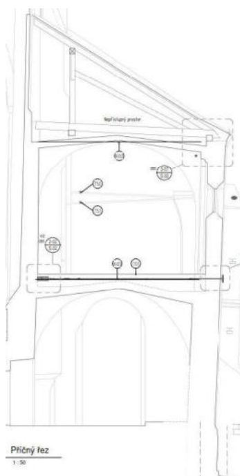
(a) Příčný řez
