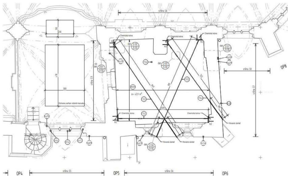
Obrázek 2: 2.np, pokladnice: Původní návrh zajištění obvodového zdiva
