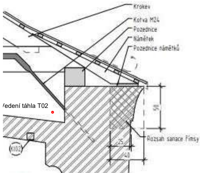
(b) Detail 3-07, poloha táhla T-02 (červeně)
