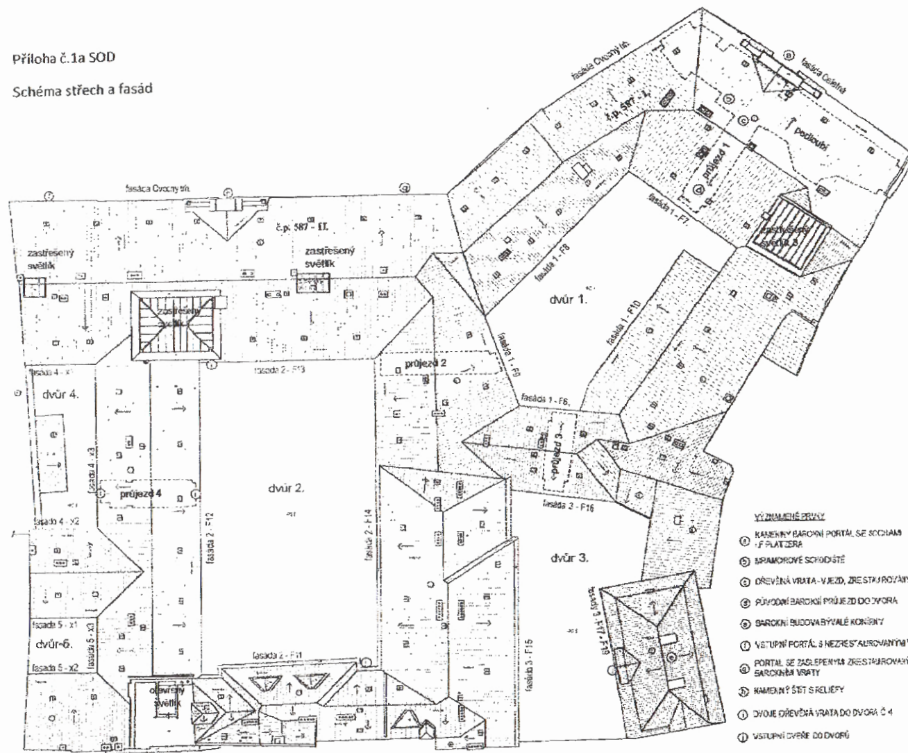
schéma střech
