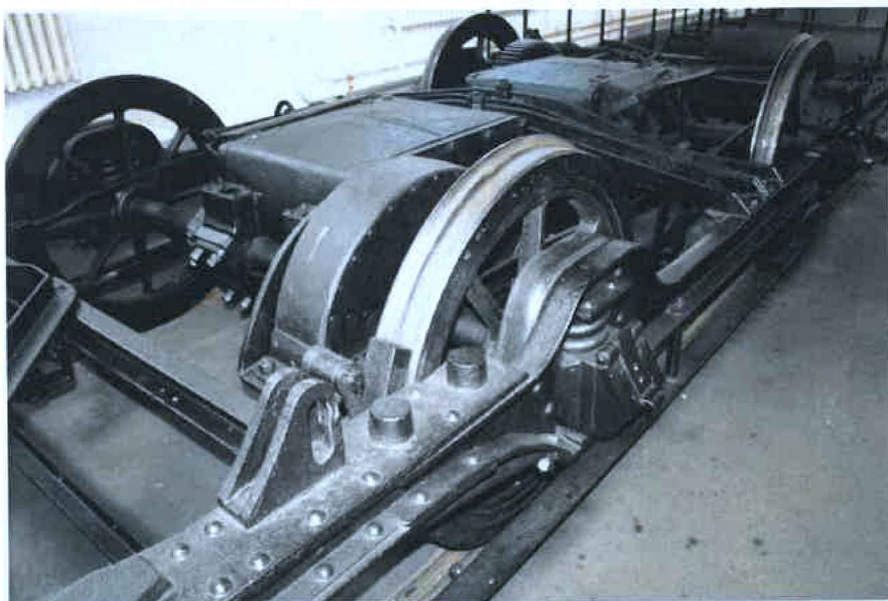
inv. č. 279 podvozek motorového vozu č. 7 Křižkovy elektrické dráhy
