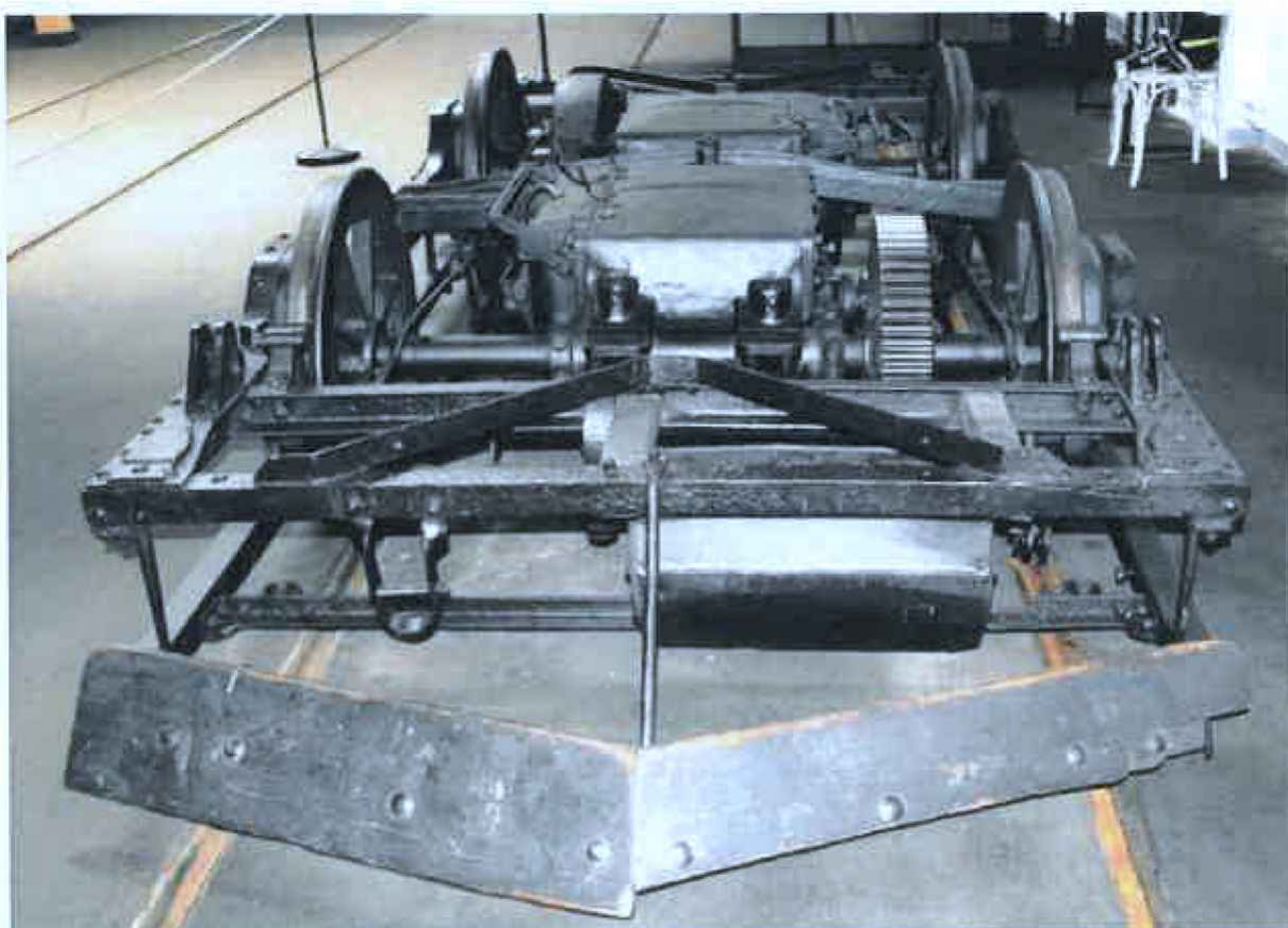
inv. č. 279 podvozek motorového vozu č. 7 Křižíkovy elektrické dráhy
