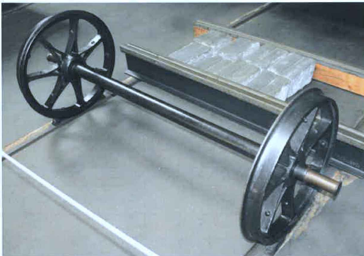
inv. č. 5038 dvojkolí z vlečného vozu pražské pouliční koňky
