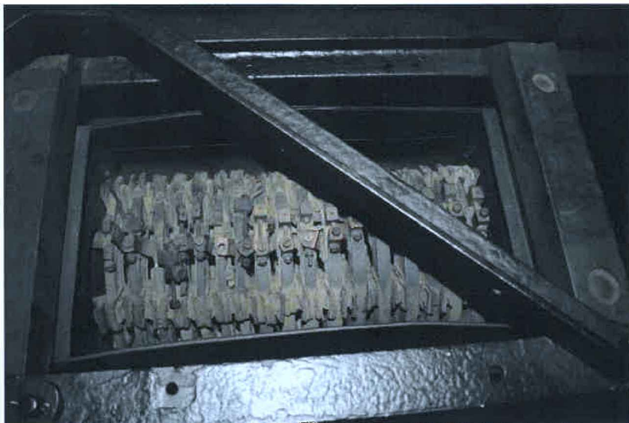
inv. č. 279 podvozek motorového vozu č. 7 Křížkovy elektrické dráhy - kontrolér
