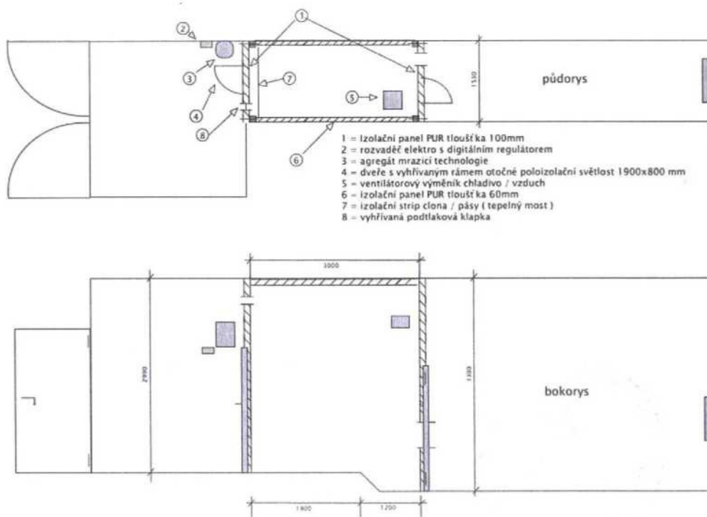
Obr. 1 – Ilustrační obrázek - Mrazicí komora pro nástřel zbraní a střeliva
