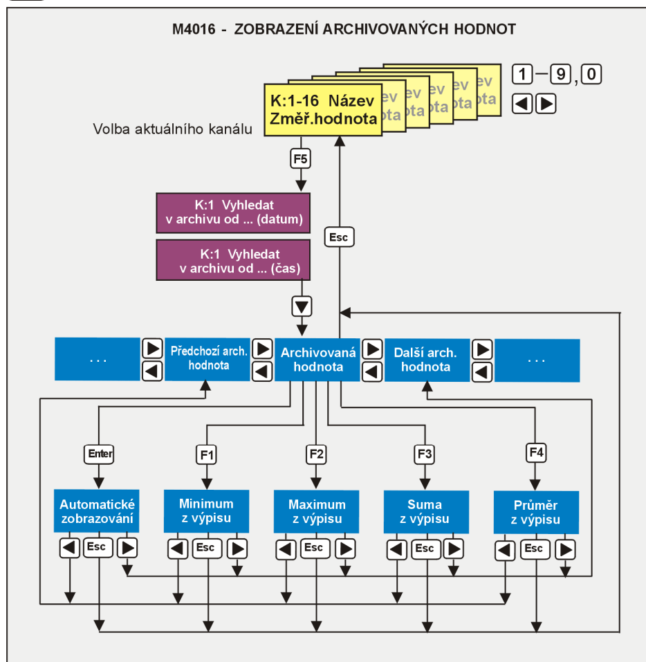
Obr. 11: Struktura služeb pro vyvolání archivovaných hodnot
