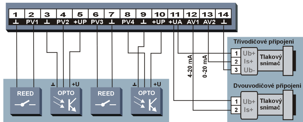
Obr. 5: Připojení snímačů k přípojné desce PPD.
