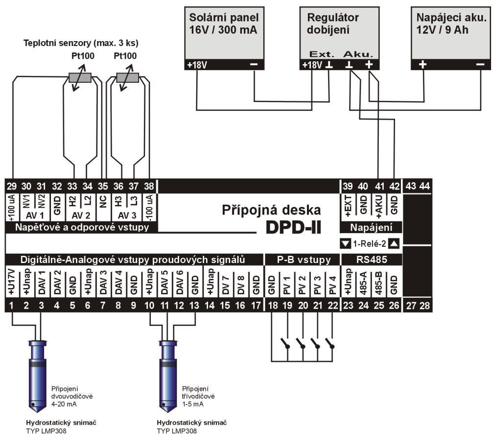
Obr. : připojení tlakových snímačů a binárních vstupů k přípojné desce DPD-II
