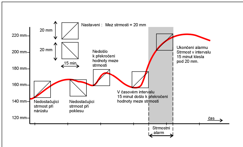
Obr. 16: Strmostní alarm
