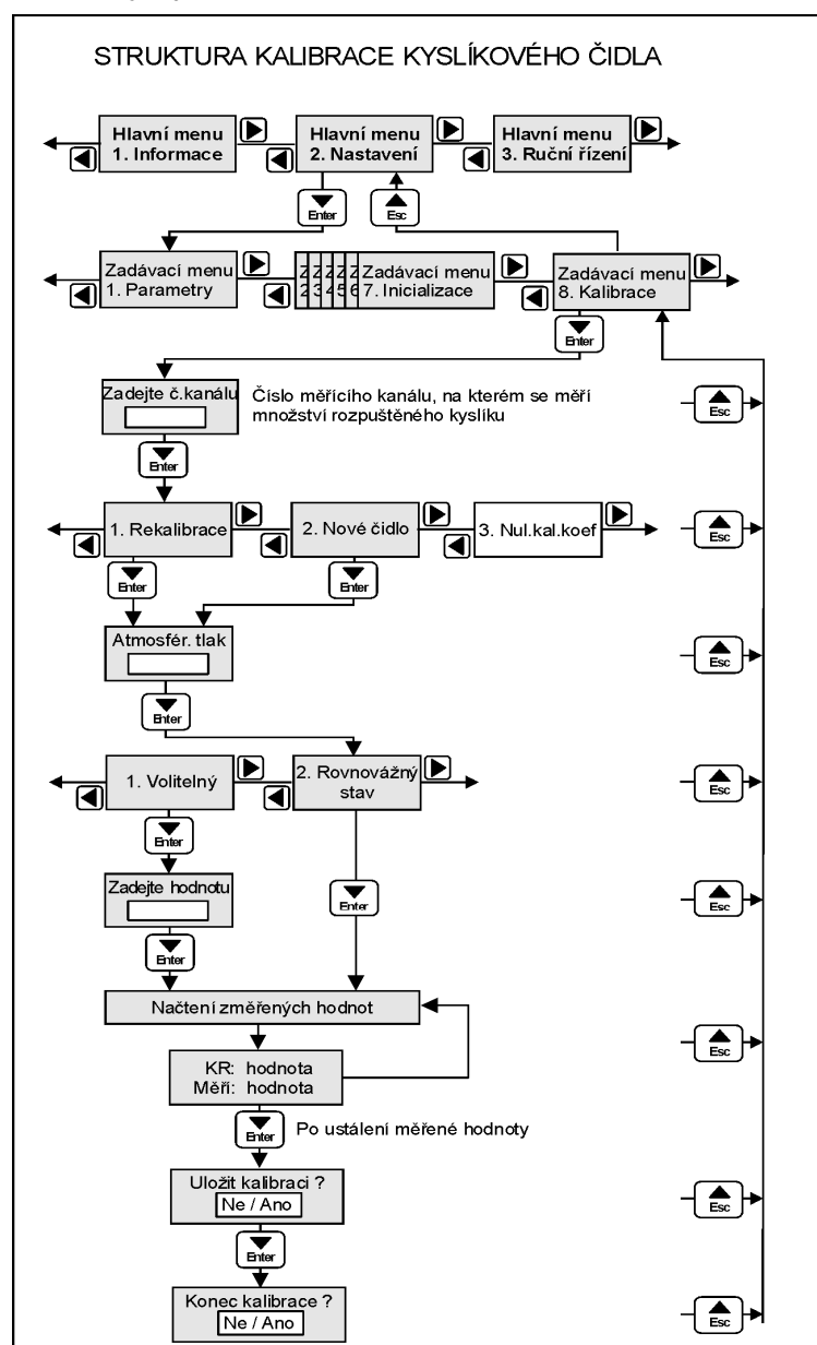
Obr. 18: Postup kalibrace kyslíkového čidla
