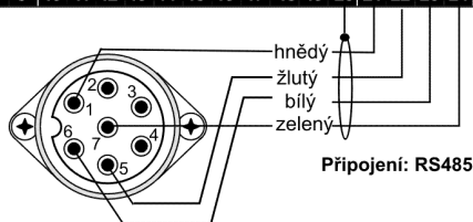
Konektor elektrochemického snímače ESK11 (ESP11, ESR11)
