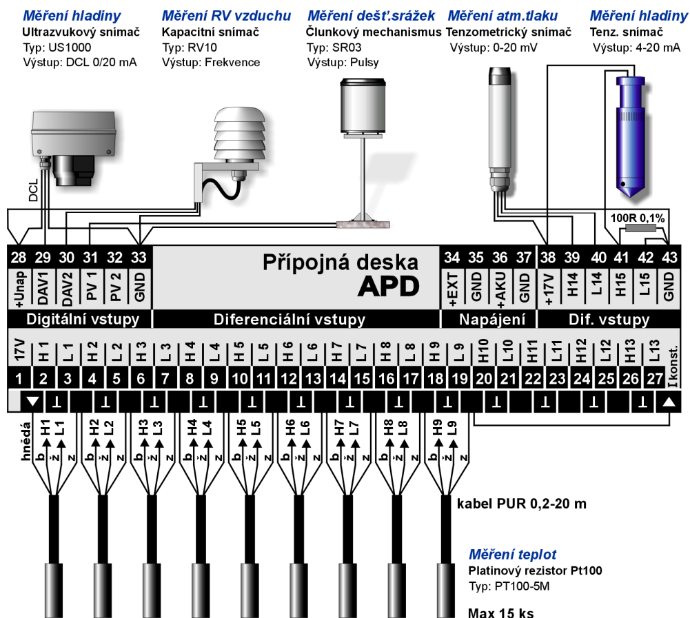
Obr. 8: Připojení různých typů snímačů k přípojné desce APD.
