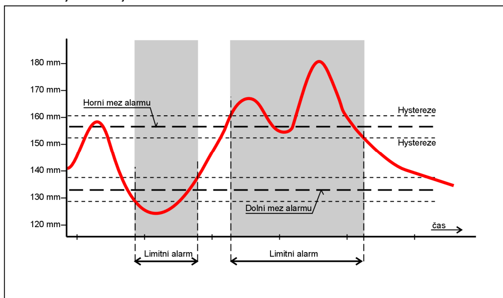
Obr. 15: Limitní alarm
