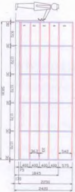
VÝKONNÉ ÚLOŽNÍ ROZVÁŽENÍ REGÁLŮ
