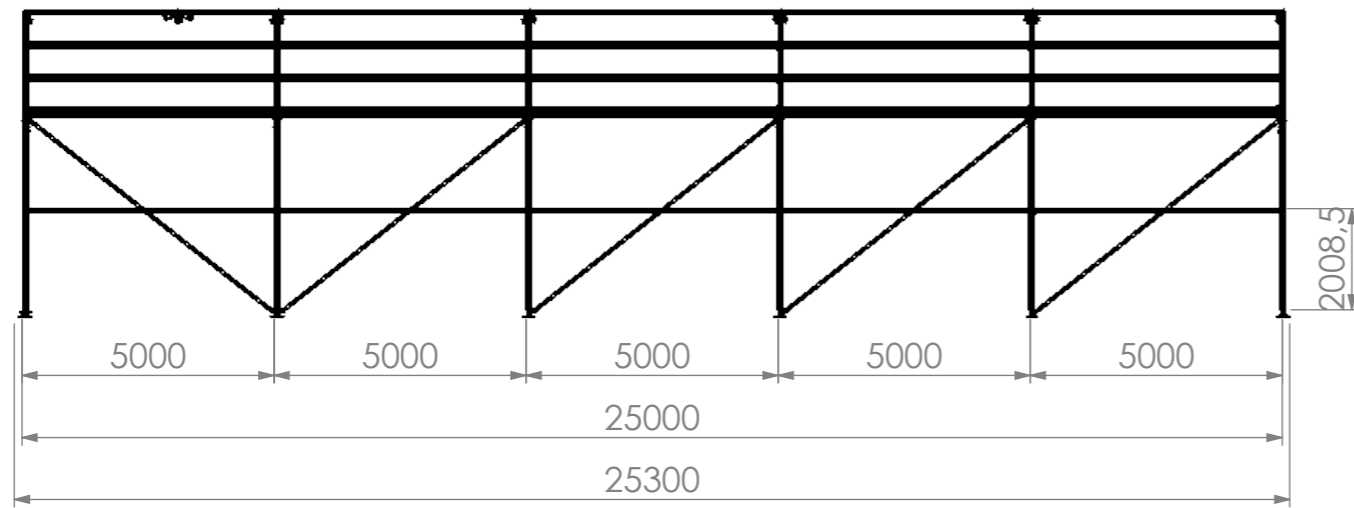
BOČNÍ POHLED
