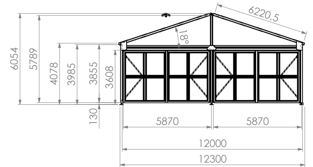
ZADNÍ POHLED
