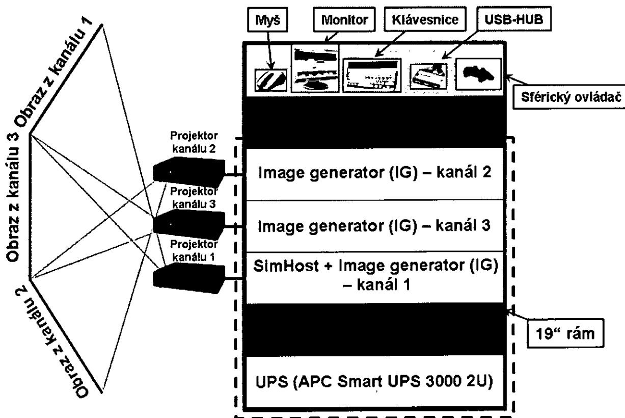
Obr. 1 – Vyobrazení složení virtuální pozorovatelny s vyznačením částí technického zhodnocení (žlutě podbarvené obdélníky)
