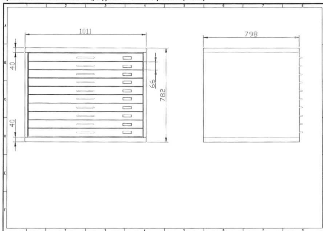
Výkresová skříň formátu A1 „atypická“ – rozměry skříně (v mm)
