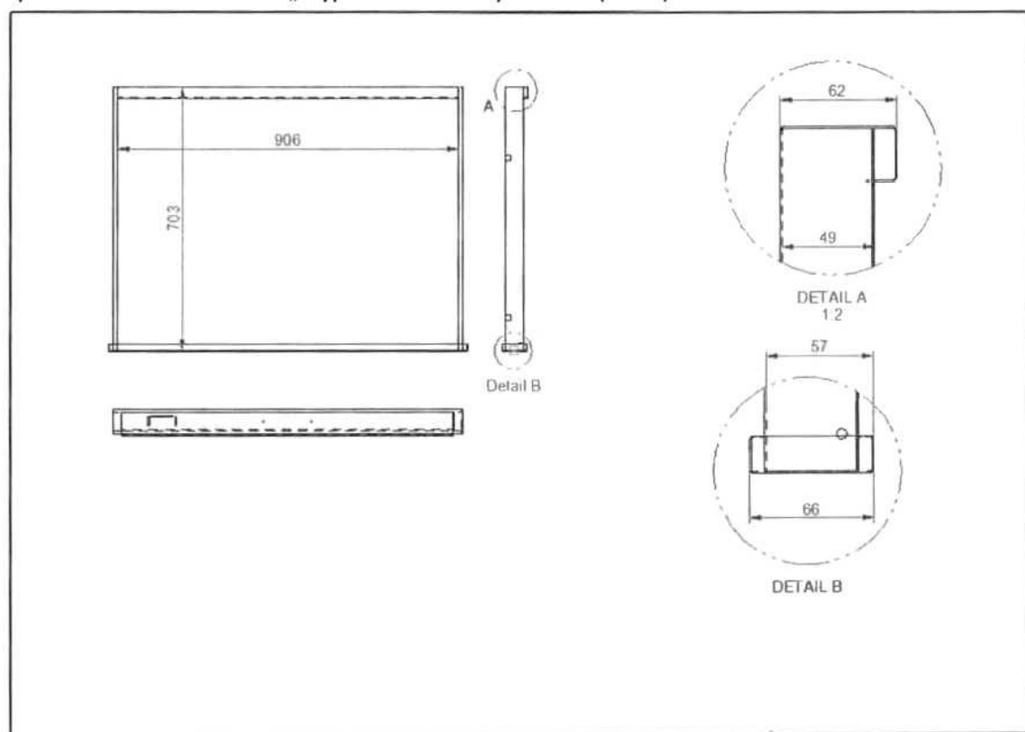
Výkresová skříň formátu A1 „atypická“ – rozměry zásuvek (v mm)
