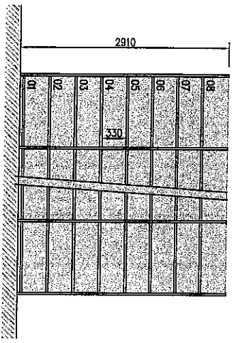
Podélný řez regálem - šanonů
