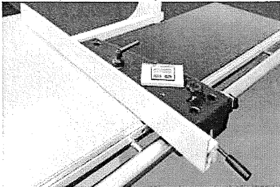
Paralelní pravítka do šířky 1000, 1.350, 1525 mm včetně digitálního odměřování (na přání)
