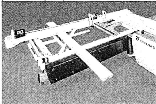
Větší výložníkový stůl s výsuvným podpěrným válečkem a digitály a kompenzací polohy pravítka (na přání)
