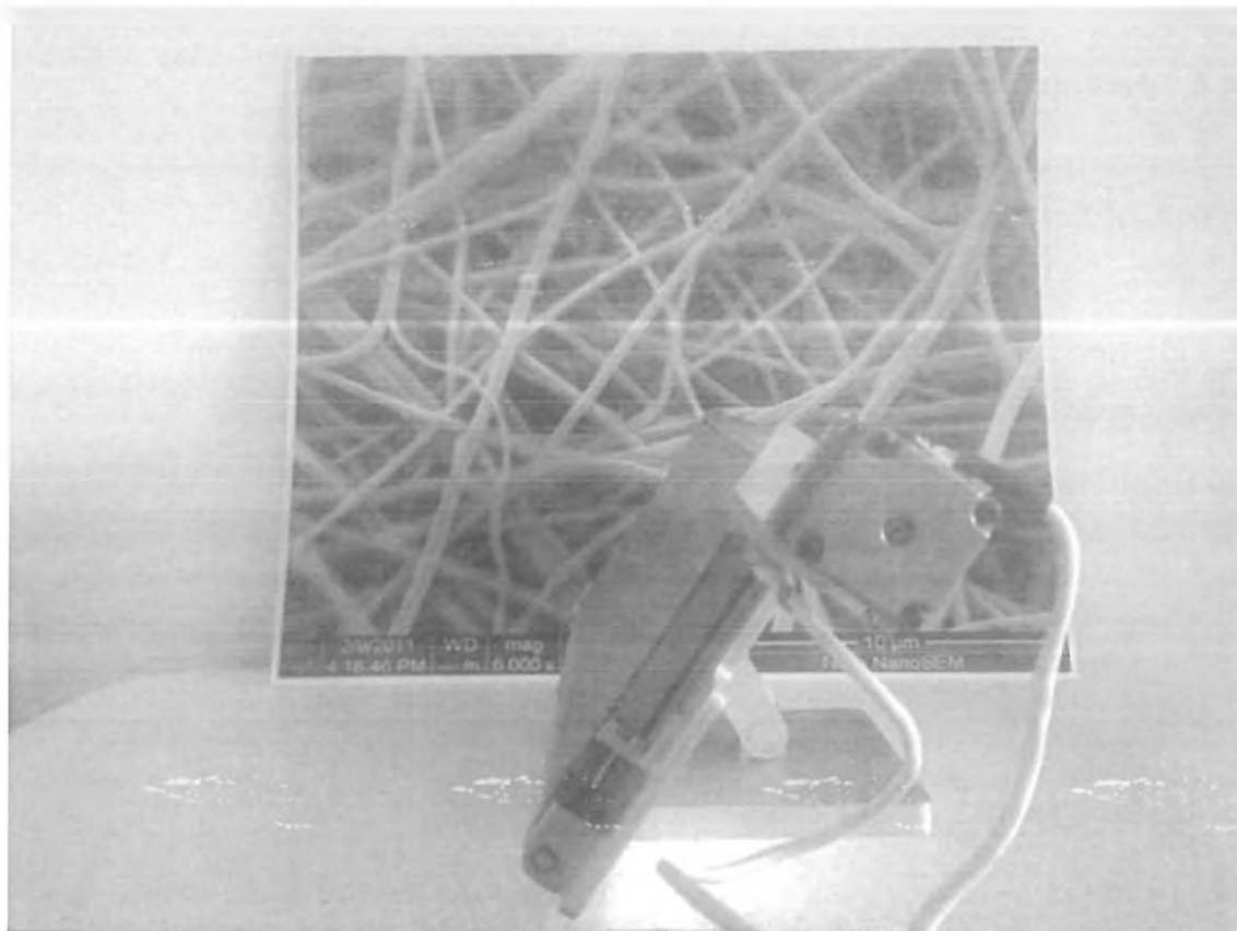
Boční pohled na depoziční jednotku
