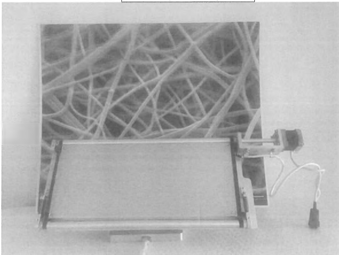
Čelní pohled na depoziční jednotku
