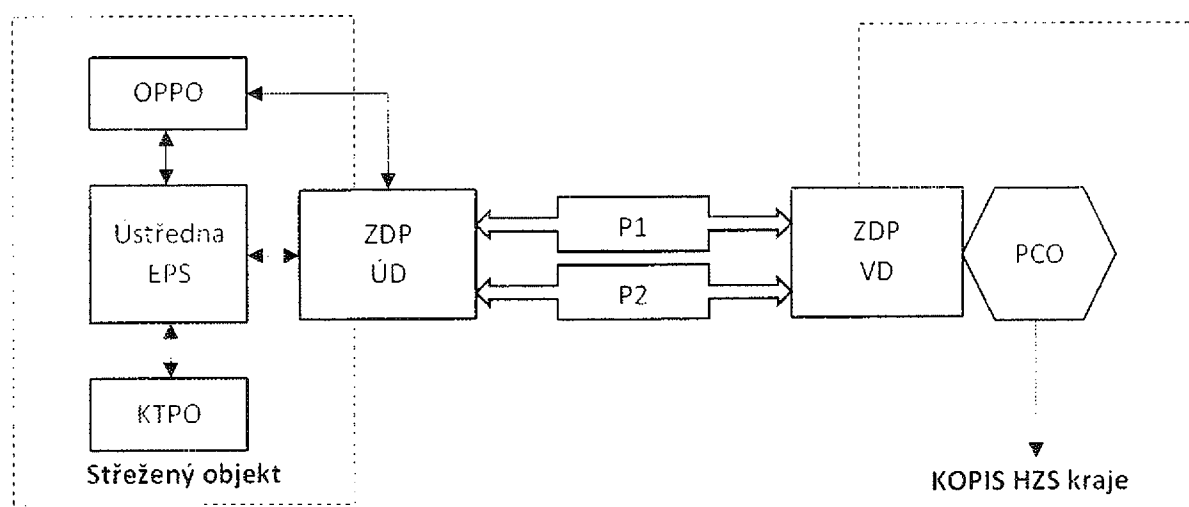
Schéma zařízení dálkového přenosu
