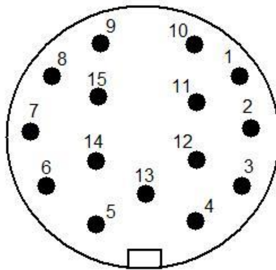
Obr.1-15 -pin zásuvka
