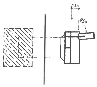
ŘEZ, 1:25
