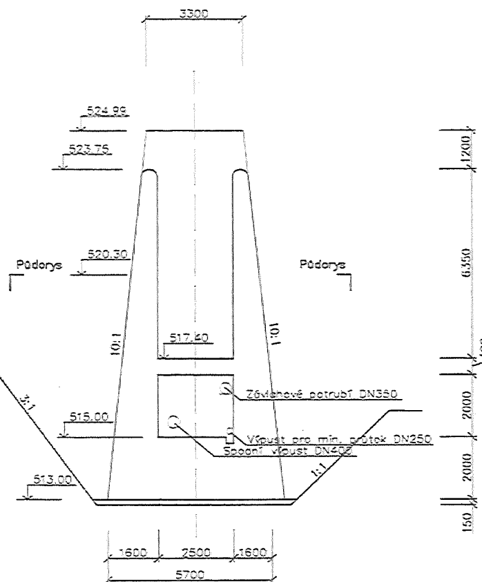
ŘEZ 2 - 2
