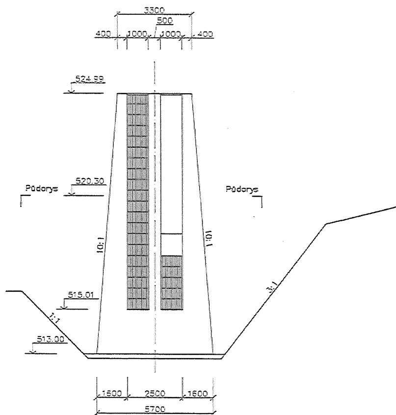
ŘEZ 1 - 1
