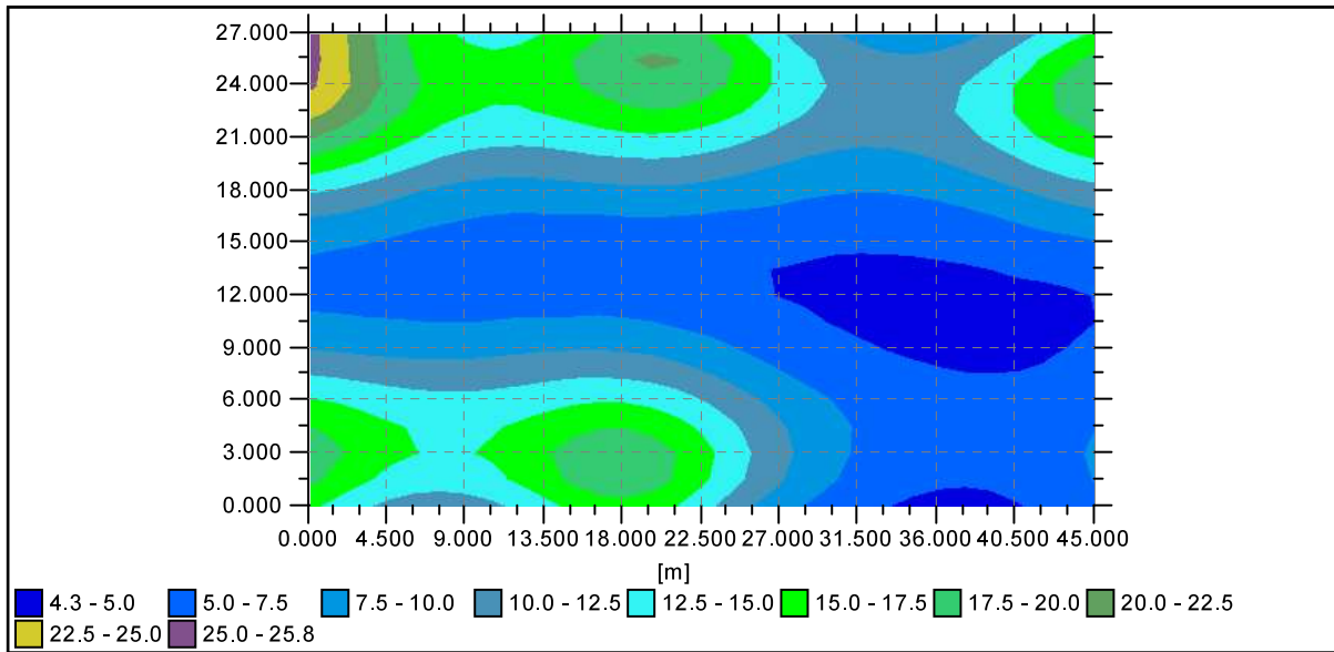
vypocetni plocha zastavka (1) : Illuminance [lux]
