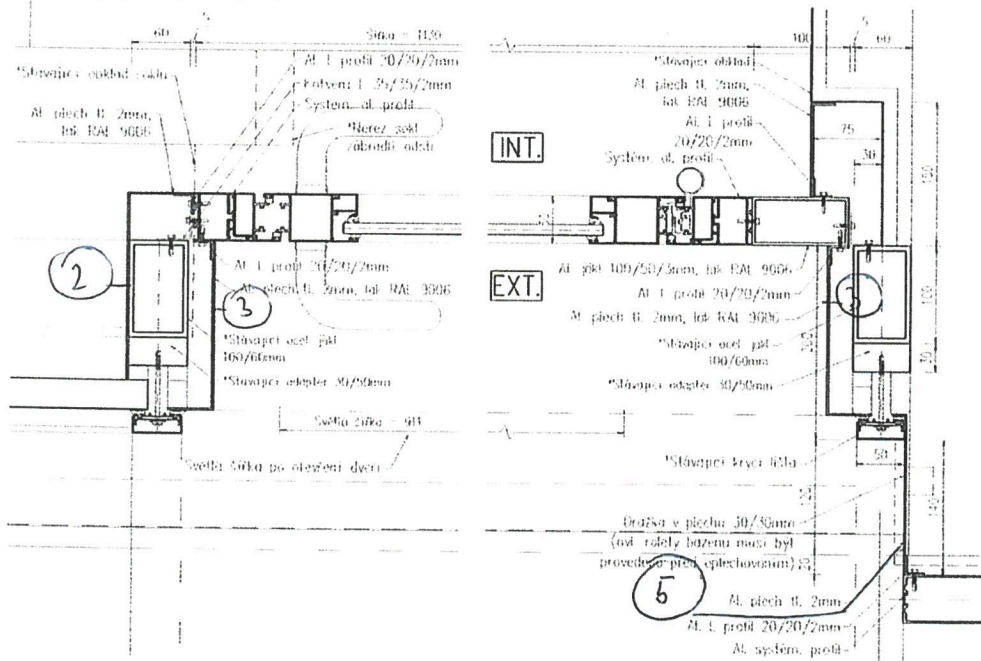
Detaily půdorysné (1:5)
