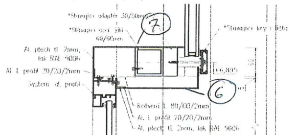
Detail svislý střed (1:5)
