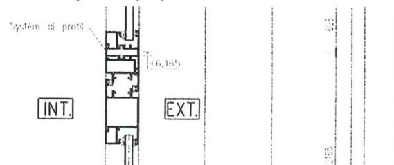
Detail svislý dole (1:5)
