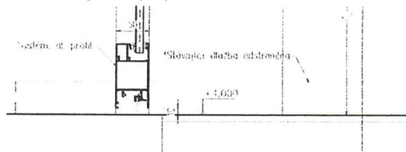
Detail svislý dole (1:5)
