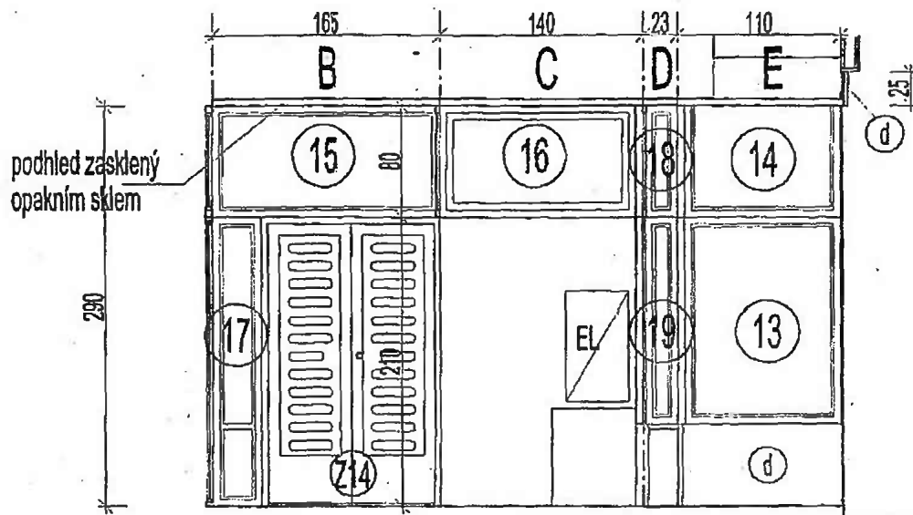
rozvinutý pohled na stěny B,C,D,E
