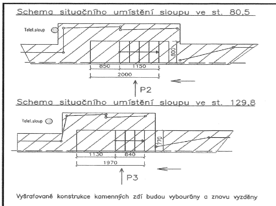
Staničení 80,5 je stávající pozice rozvodného sloupu
