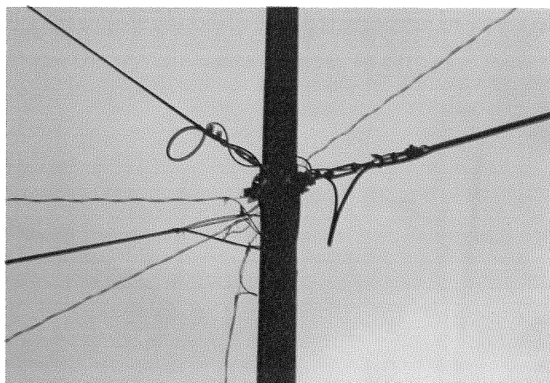
Objímka s kabely na rozvodném sloupu
