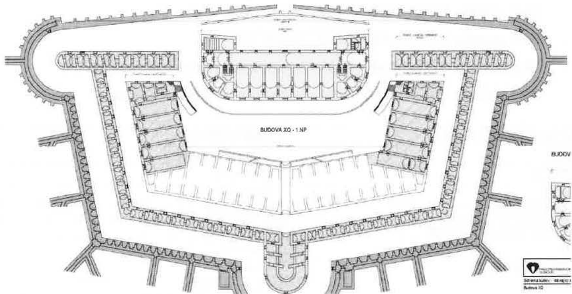
Půdorysné schéma, reduit žlutě.
