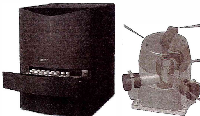
Obr. 1. Ilustrační obrázek systému LSC HIDEX 300 SL a uspořádání měřicí komory se 3 fotonásobiči
