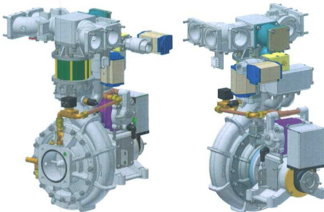
Ilustrační 3D Model čerpadla PKA 2000 -250
