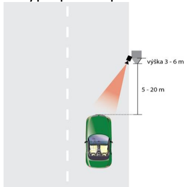
Schéma instalace kamery pro správné rozpoznávání SPZ
