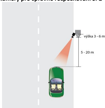
Schéma instalace kamery pro správné rozpoznávání SPZ
