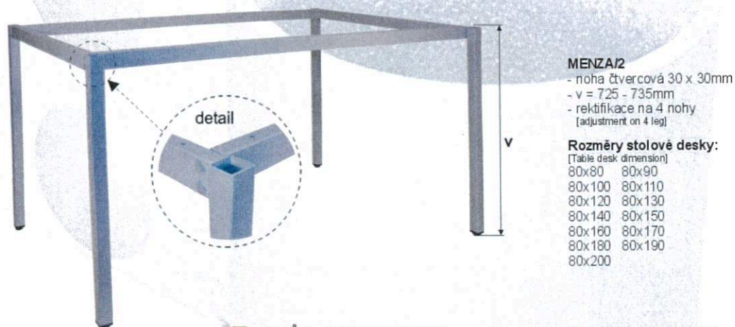
■ STŮL "MENZA/2" - noha čtvercová 30 x 30mm [TABLE "MENZA/2" - SQUARE LEG 30 x 30mm]
