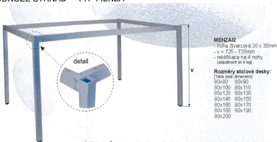
■ STŮL "MENZA/2" - noha čtvercová 30 x 30mm [TABLE "MENZA/2" - SQUARE LEG 30 x 30mm]
