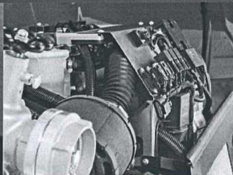
Elektronický systém vstřikování se snadno přístupným rozhraním OBD
