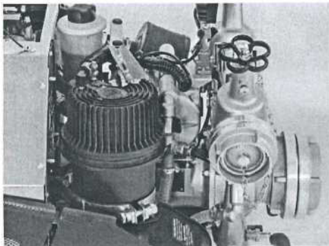
Vodou chlazený dvouválcový 4taktní benzínový motor se suchou klikovou skříní
