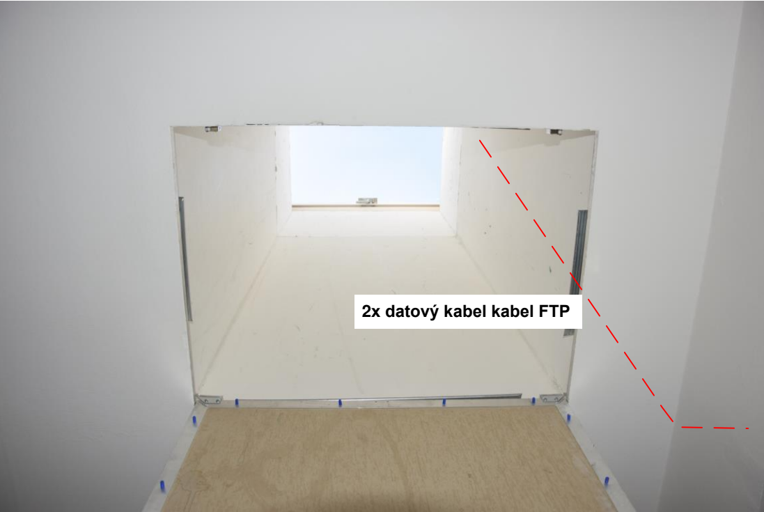
11. Místnost 2.10 WC - kabelová trasa ze střechy do technologické skřínky
