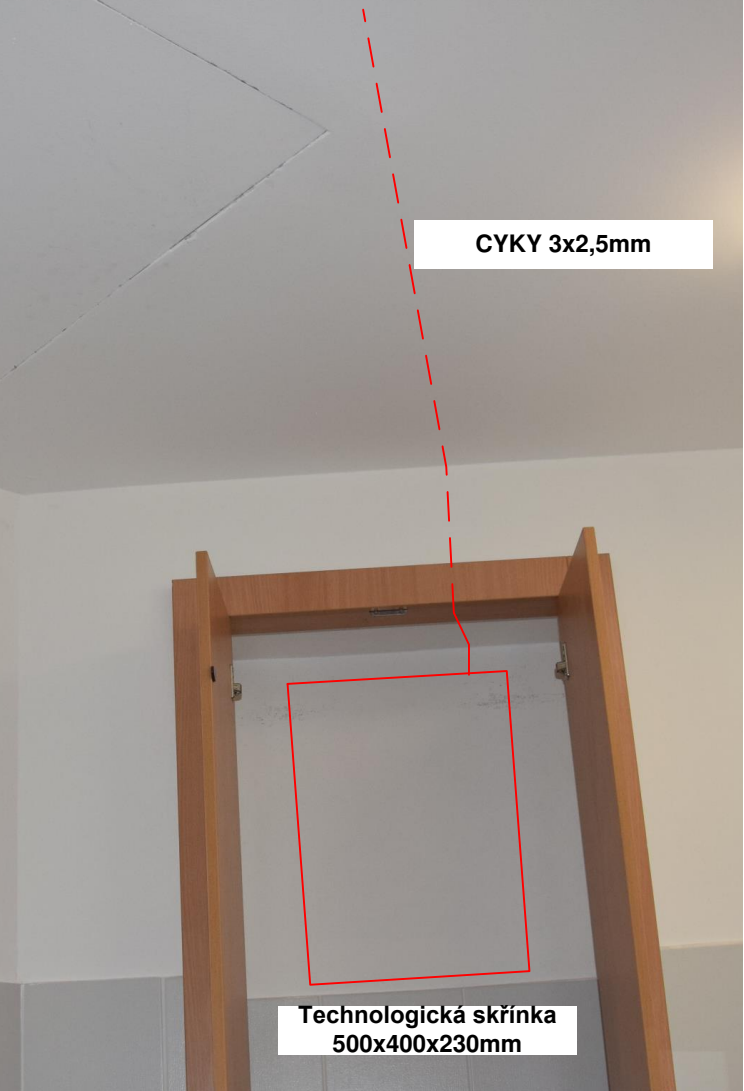
9. 2NP místnost 2.10 Umístění technologické skřínky ve falešné skříně.
