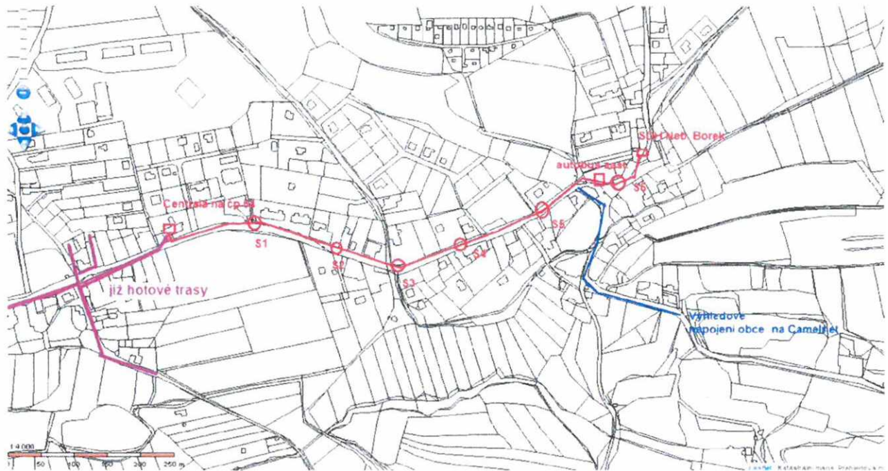
Obr. Schéma optické sítě Nebílovský Borek
