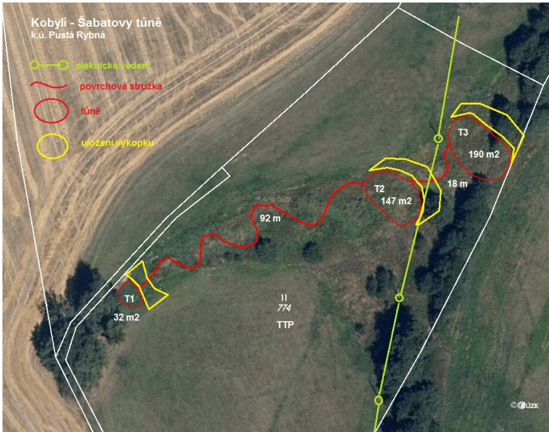
Obr. 4 Situace kácení
