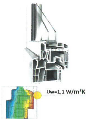
Dvojitě zasklení 24 mm Hliníkový distanční rámeček
