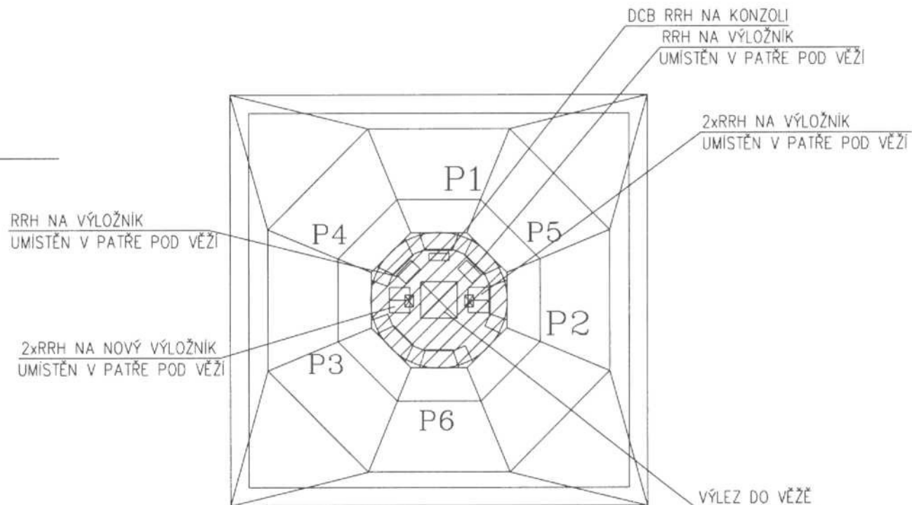
ROZMÍSTĚNÍ ANTÉN
